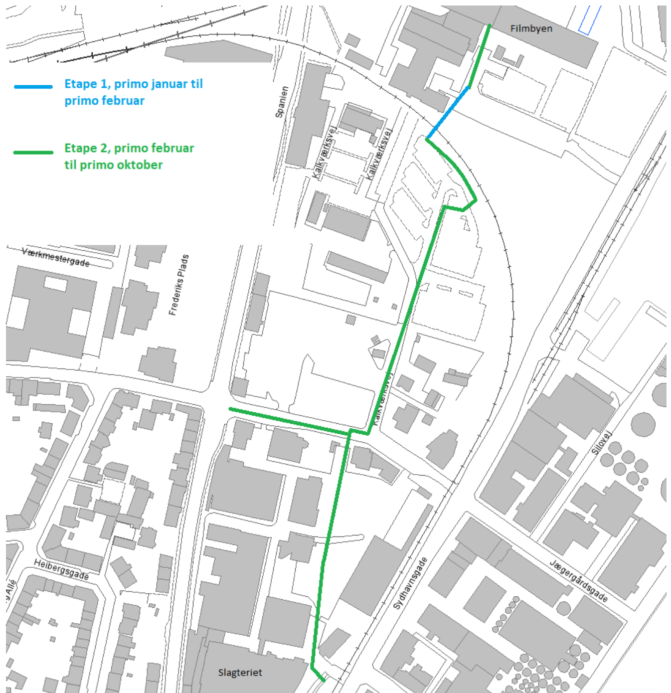
billede 1: Fjernvarmetrace
